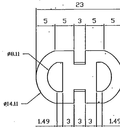
C-C
