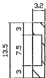
B-B
