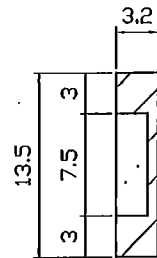
B-B
