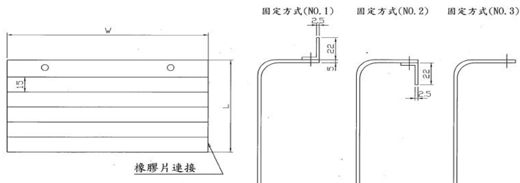
鋁合金防護簾(二)橡膠
