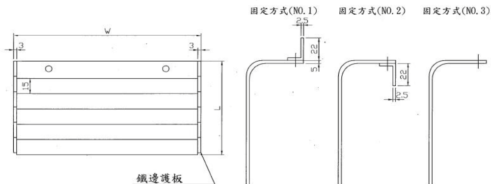
鋁合金防護簾(一)鐵邊
